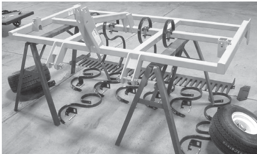
Fig. 11 - Lay-out
